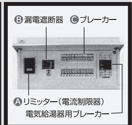
電気給湯器用ブレーカー有の分電盤
