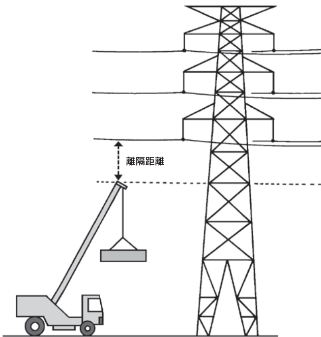
送電線から離すべき距離(離隔距離)
