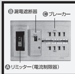
分電盤
